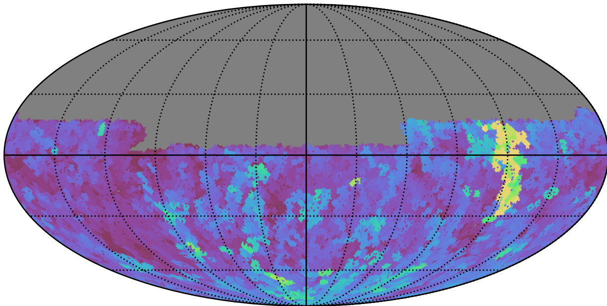
no_long_daily_v3.4_10yrs Yr1 u band: Max seeingGeom
