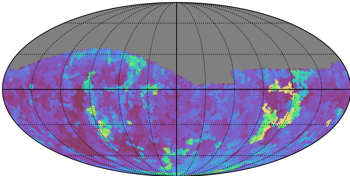
no_long_daily_v3.4_10yrs Yr1 g band: Max seeingGeom
