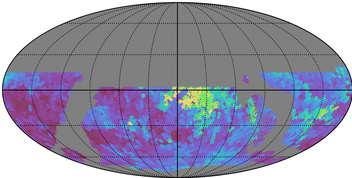
no_long_daily_v3.4_10yrs WFD y band: Max seeingEff
