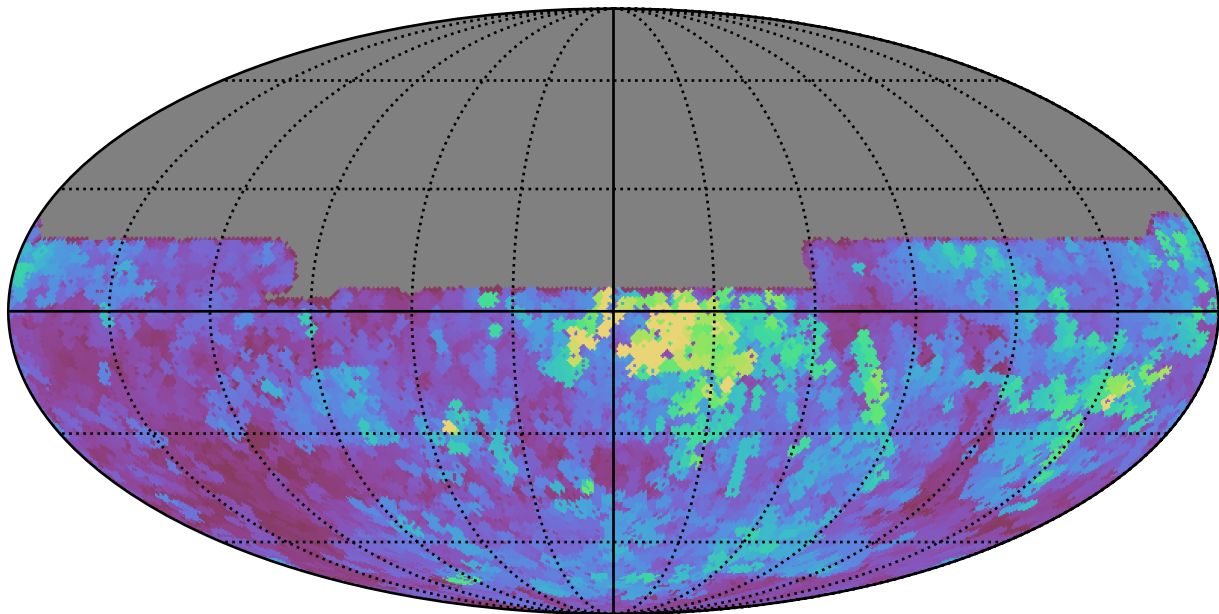
no_long_daily_v3.4_10yrs All sky y band: Max seeingEff
