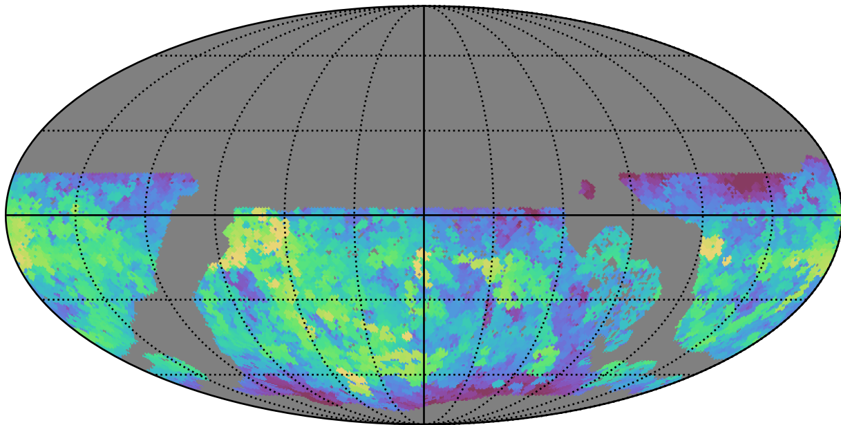
no_long_daily_v3.4_10yrs WFD g band: Max saturation_mag
