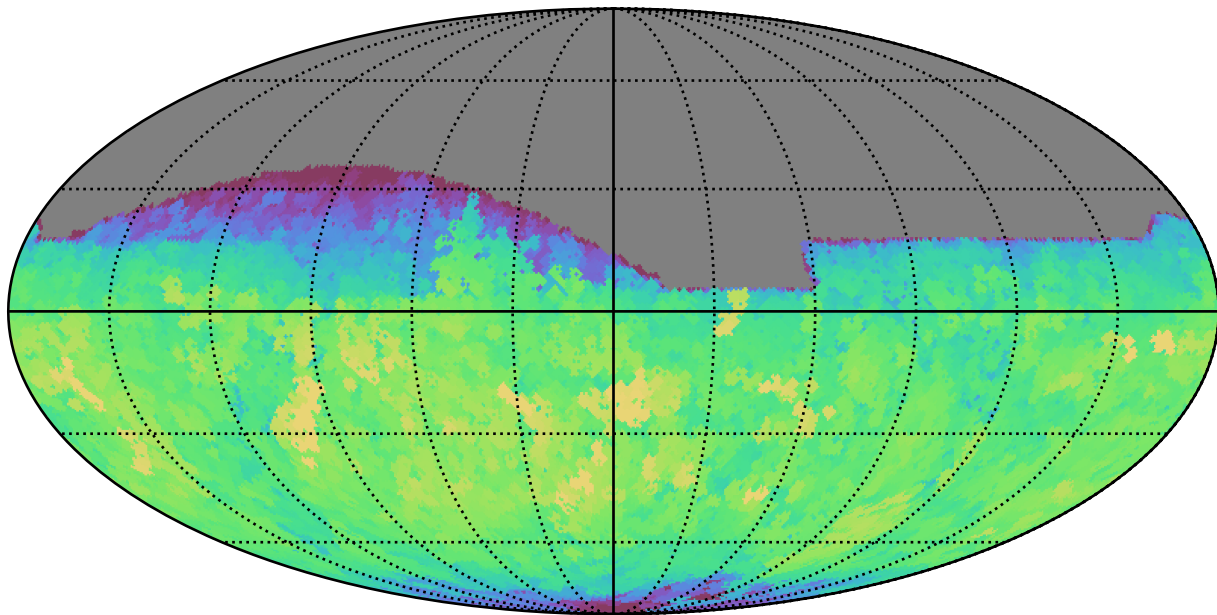
no_long_daily_v3.4_10yrs All sky z band: Max saturation_mag
