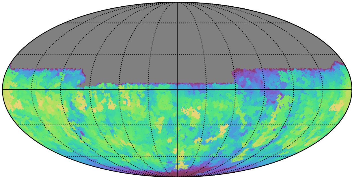
no_long_daily_v3.4_10yrs All sky u band: Max saturation_mag
