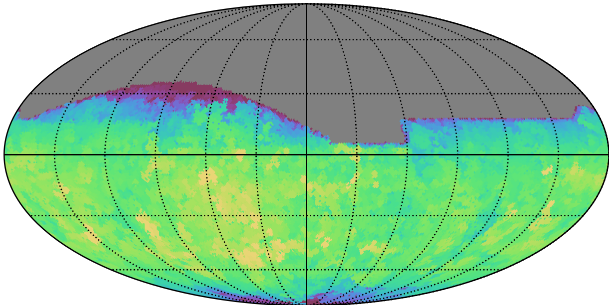
no_long_daily_v3.4_10yrs All sky r band: Max saturation_mag
