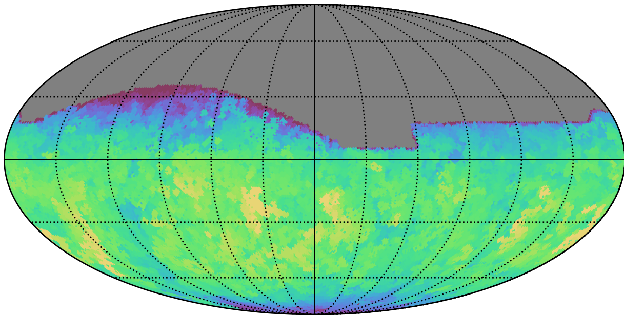
no_long_daily_v3.4_10yrs All sky i band: Max saturation_mag
