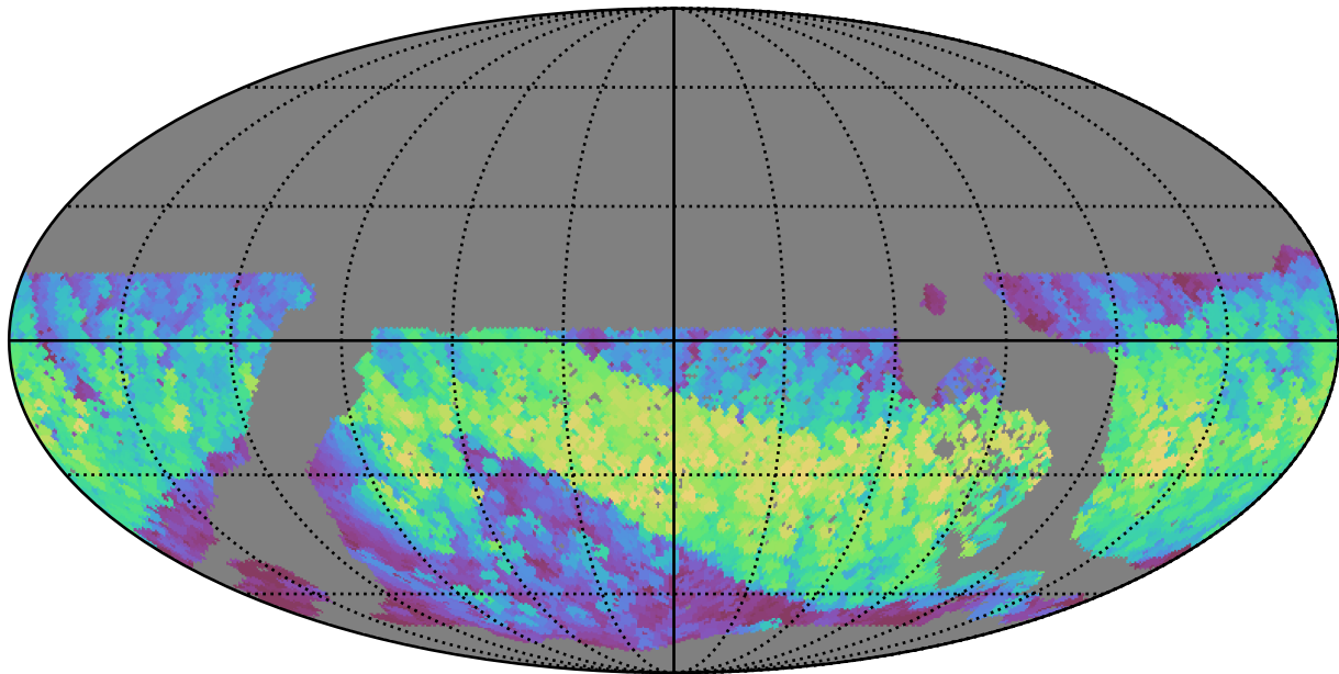
no_long_daily_v3.4_10yrs WFD z band: Max normairmass
