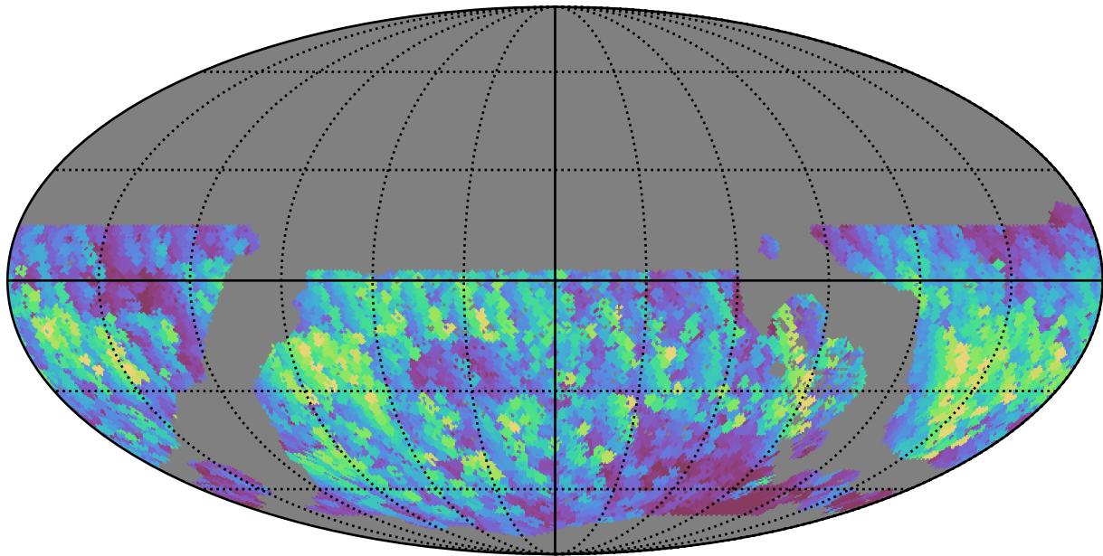
no_long_daily_v3.4_10yrs WFD y band: Max normairmass
