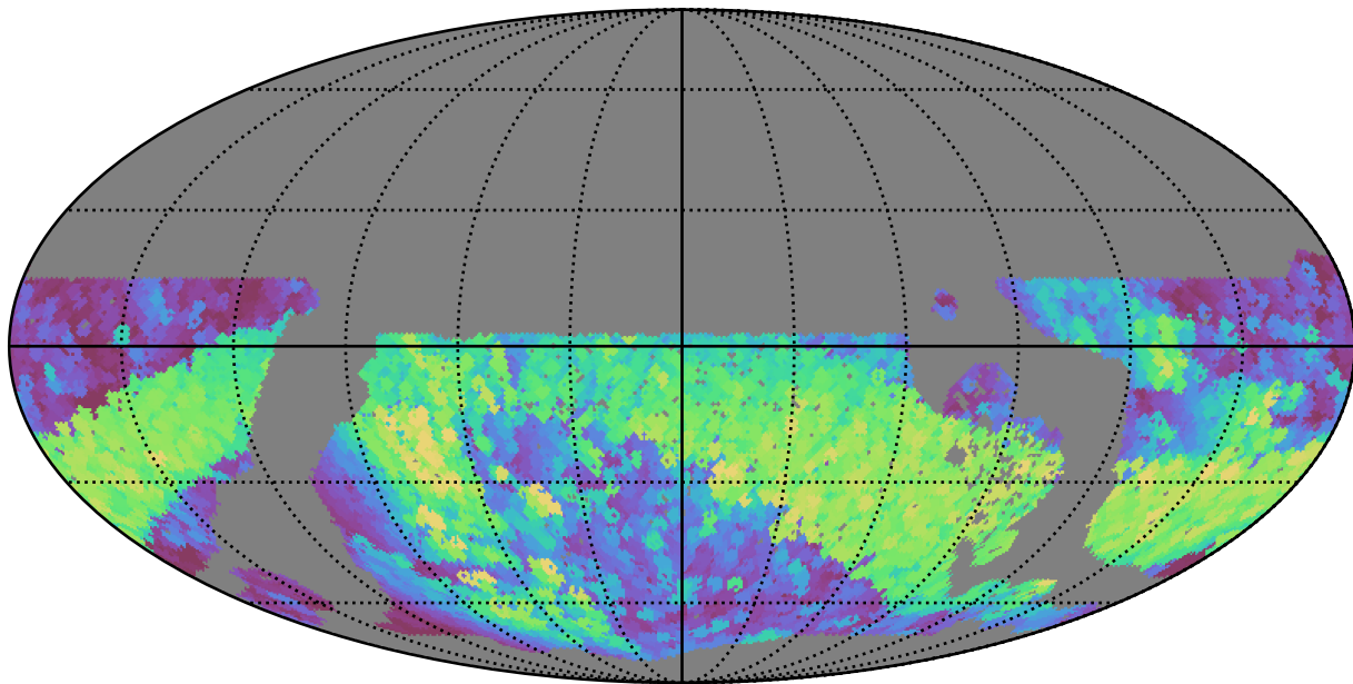
no_long_daily_v3.4_10yrs WFD r band: Max normairmass
