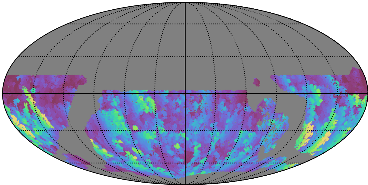
no_long_daily_v3.4_10yrs WFD g band: Max normairmass
