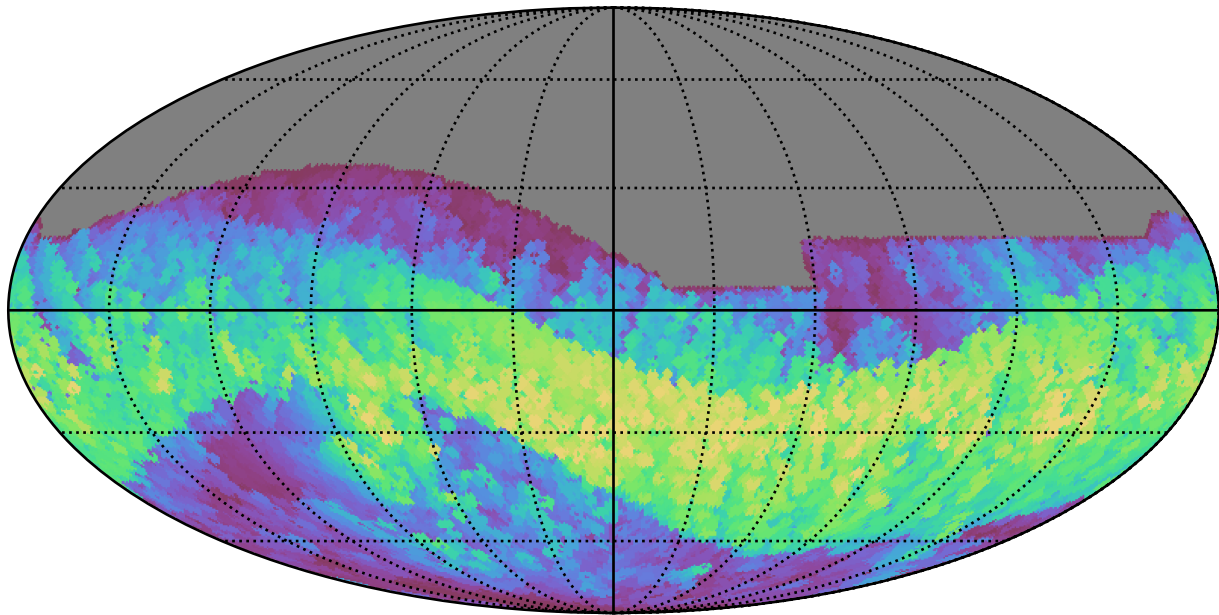
no_long_daily_v3.4_10yrs All sky z band: Max normairmass
