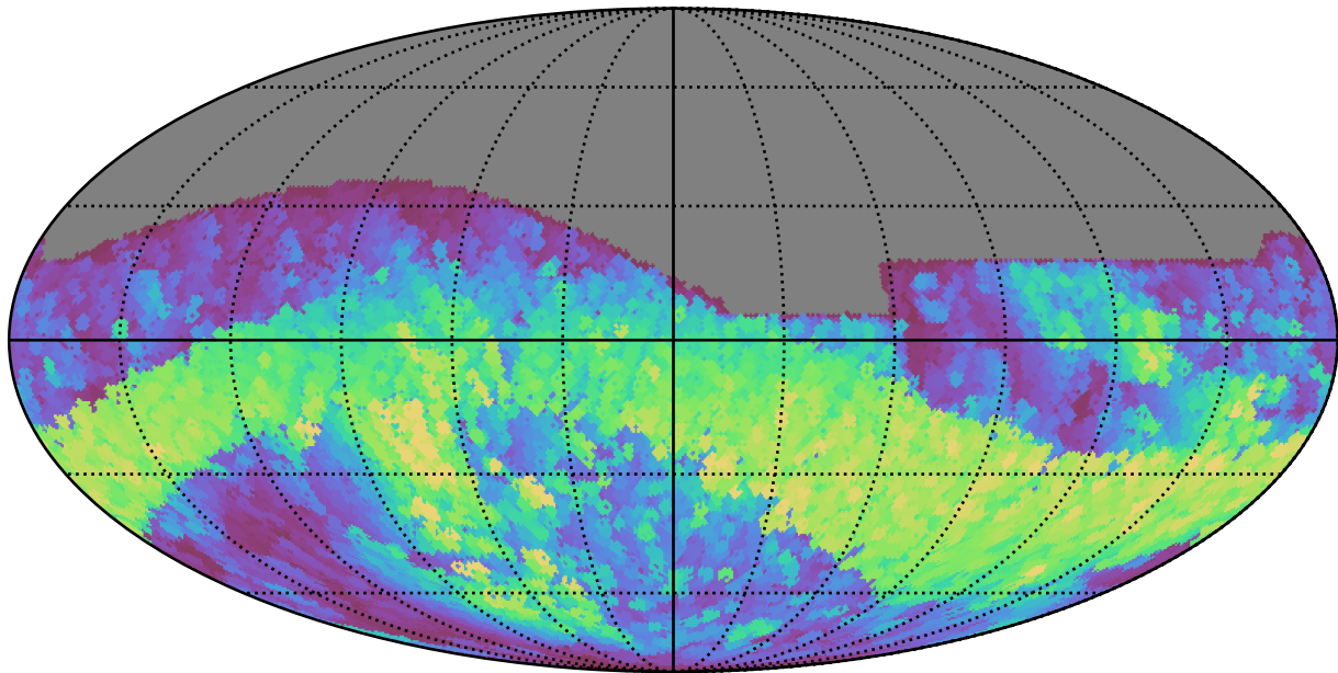
no_long_daily_v3.4_10yrs All sky r band: Max normairmass
