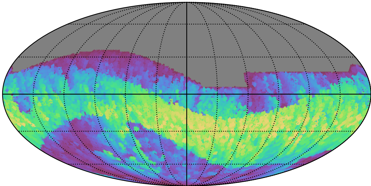
no_long_daily_v3.4_10yrs All sky i band: Max normairmass
