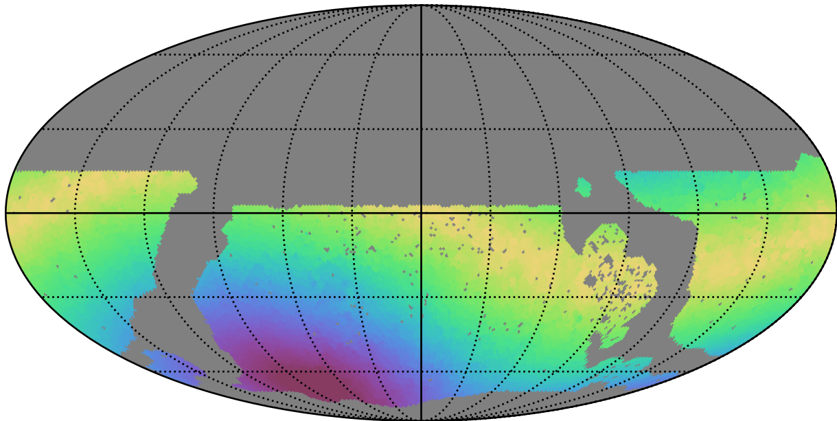
no_long_daily_v3.4_10yrs WFD i band: Max moonDistance
