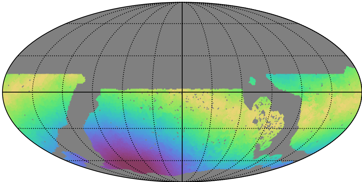
no_long_daily_v3.4_10yrs WFD g band: Max moonDistance
