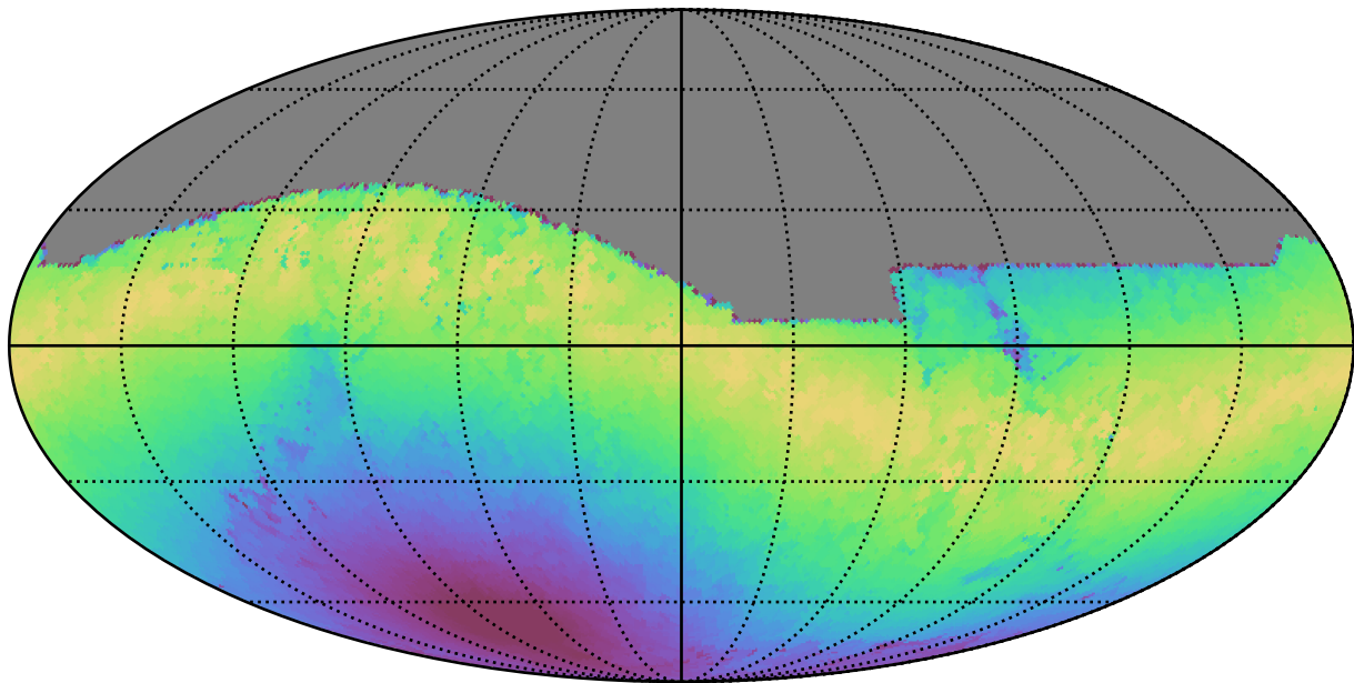
no_long_daily_v3.4_10yrs All sky z band: Max moonDistance
