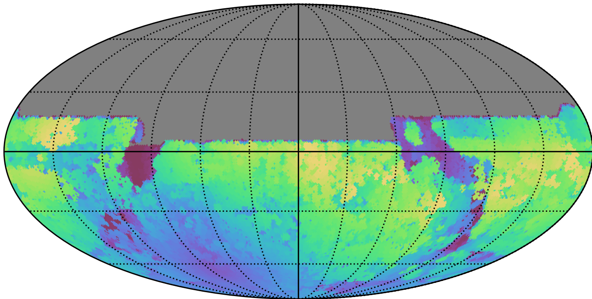
no_long_daily_v3.4_10yrs All sky y band: Max moonDistance
