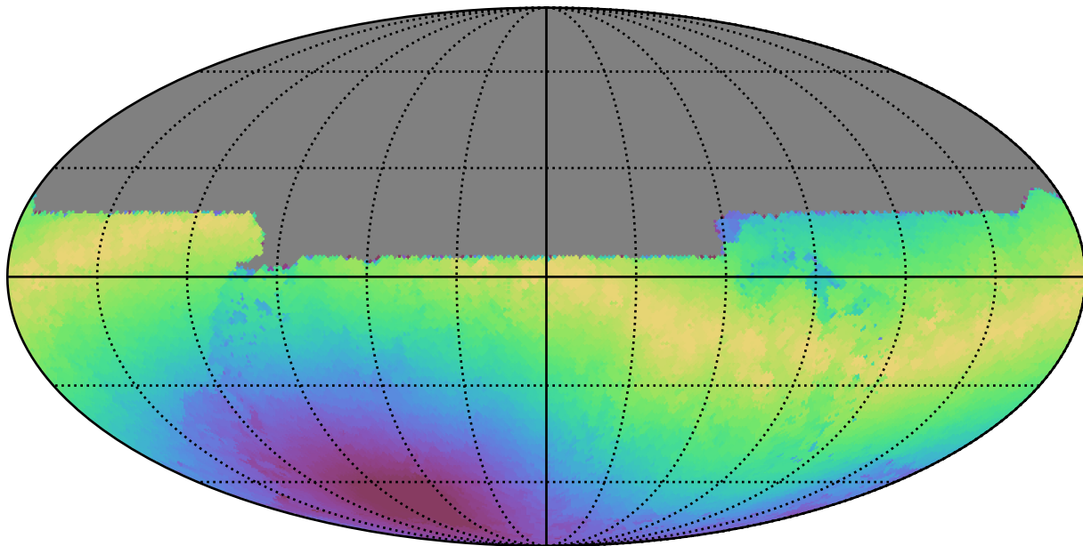
no_long_daily_v3.4_10yrs All sky u band: Max moonDistance
