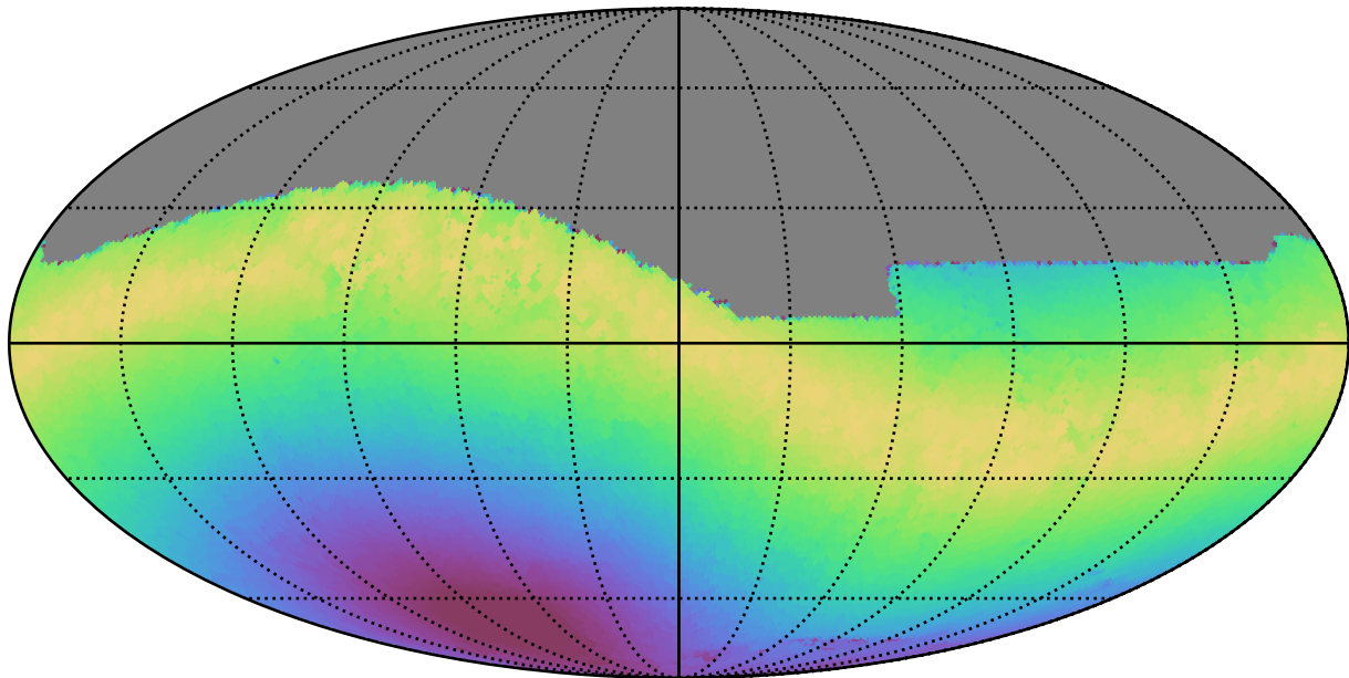
no_long_daily_v3.4_10yrs All sky r band: Max moonDistance
