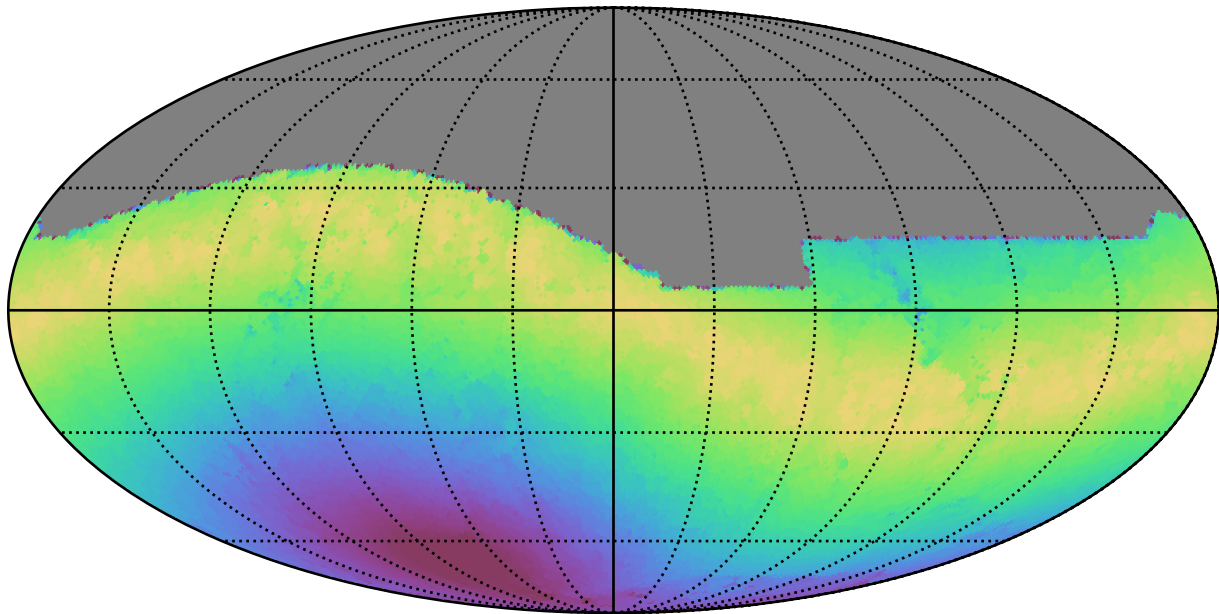
no_long_daily_v3.4_10yrs All sky i band: Max moonDistance
