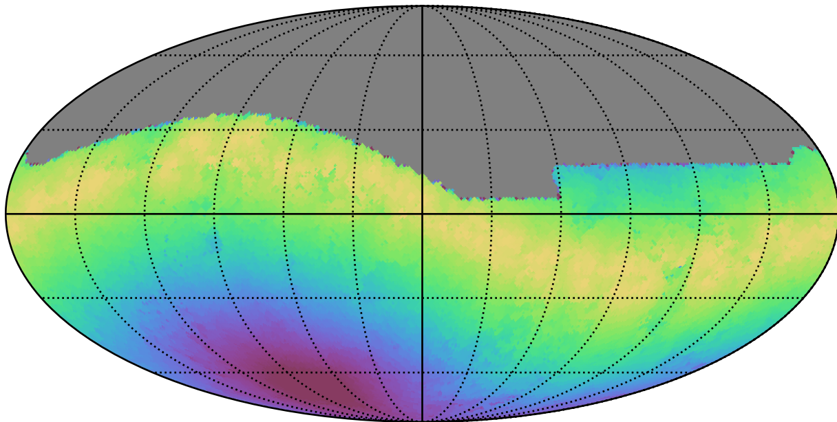
no_long_daily_v3.4_10yrs All sky g band: Max moonDistance
