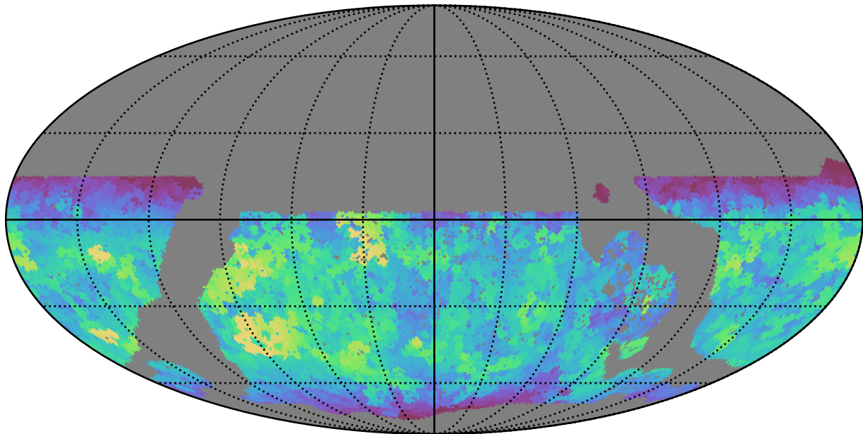
no_long_daily_v3.4_10yrs WFD y band: Max fiveSigmaDepth
