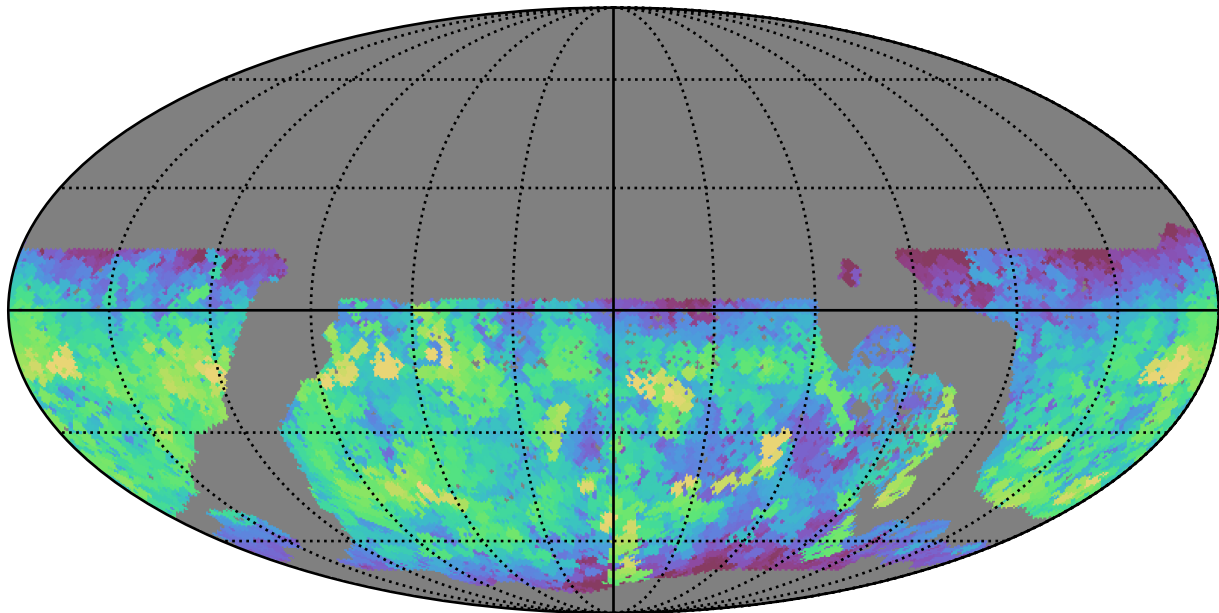
no_long_daily_v3.4_10yrs WFD u band: Max fiveSigmaDepth
