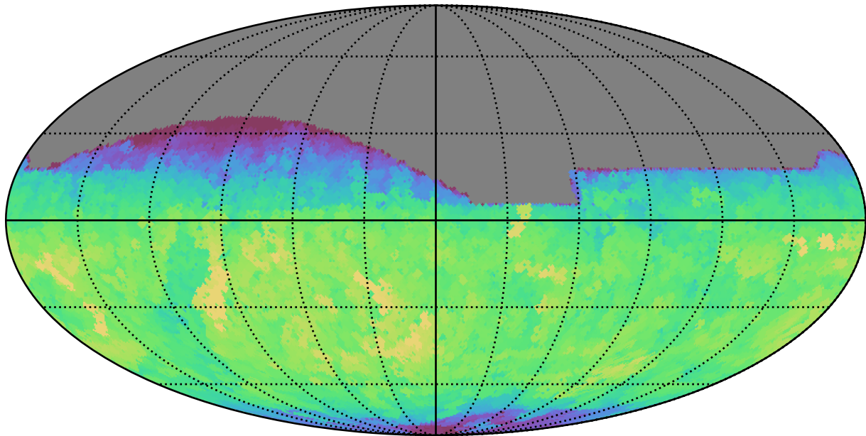
no_long_daily_v3.4_10yrs All sky z band: Max fiveSigmaDepth
