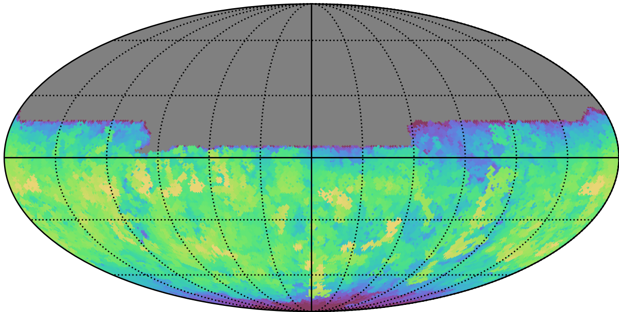
no_long_daily_v3.4_10yrs All sky u band: Max fiveSigmaDepth
