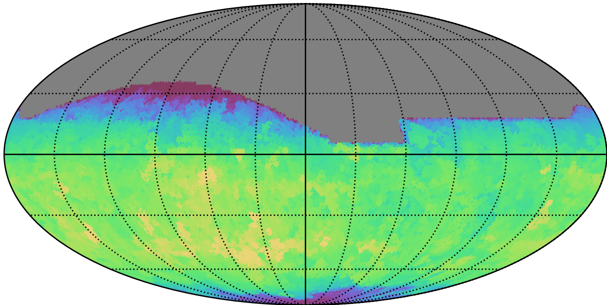
no_long_daily_v3.4_10yrs All sky r band: Max fiveSigmaDepth
