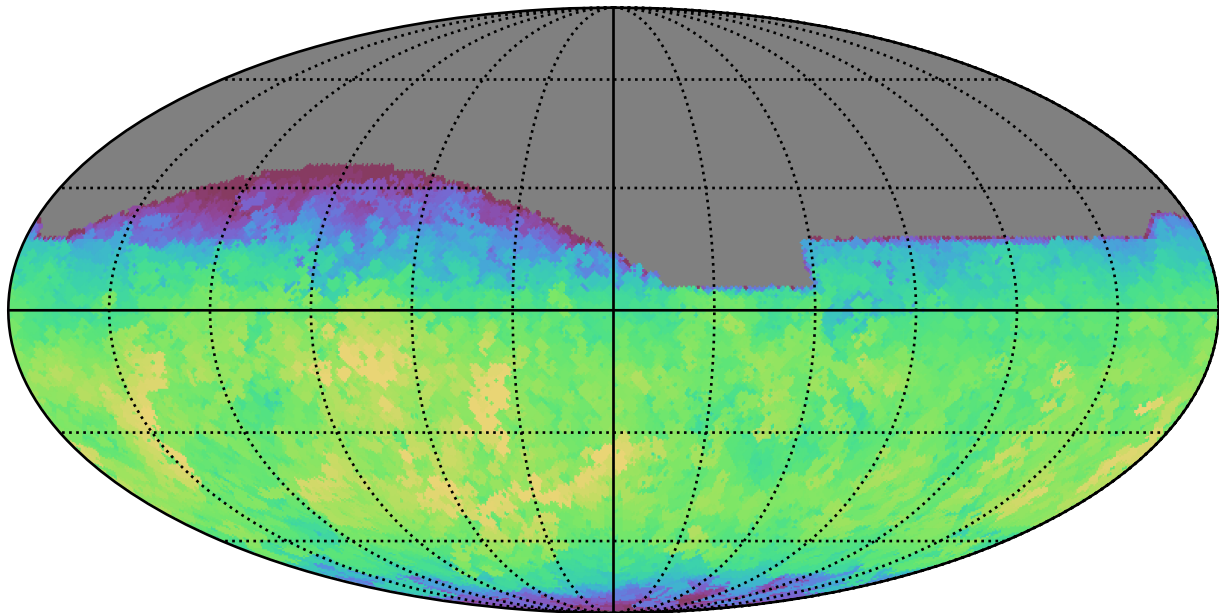
no_long_daily_v3.4_10yrs All sky i band: Max fiveSigmaDepth
