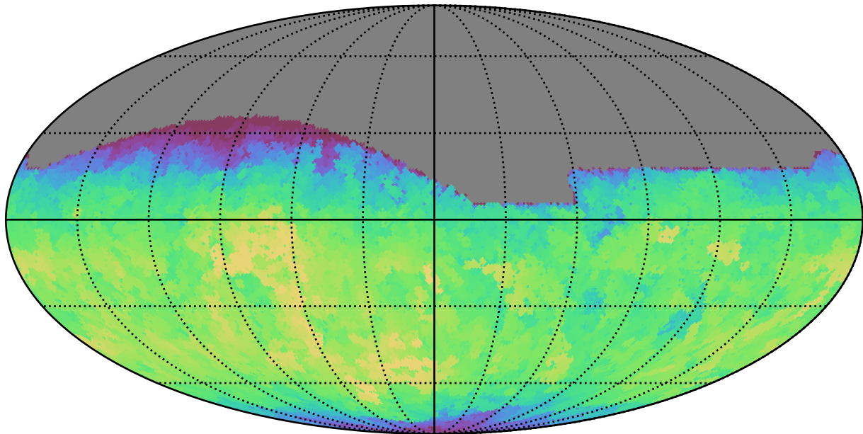
no_long_daily_v3.4_10yrs All sky g band: Max fiveSigmaDepth
