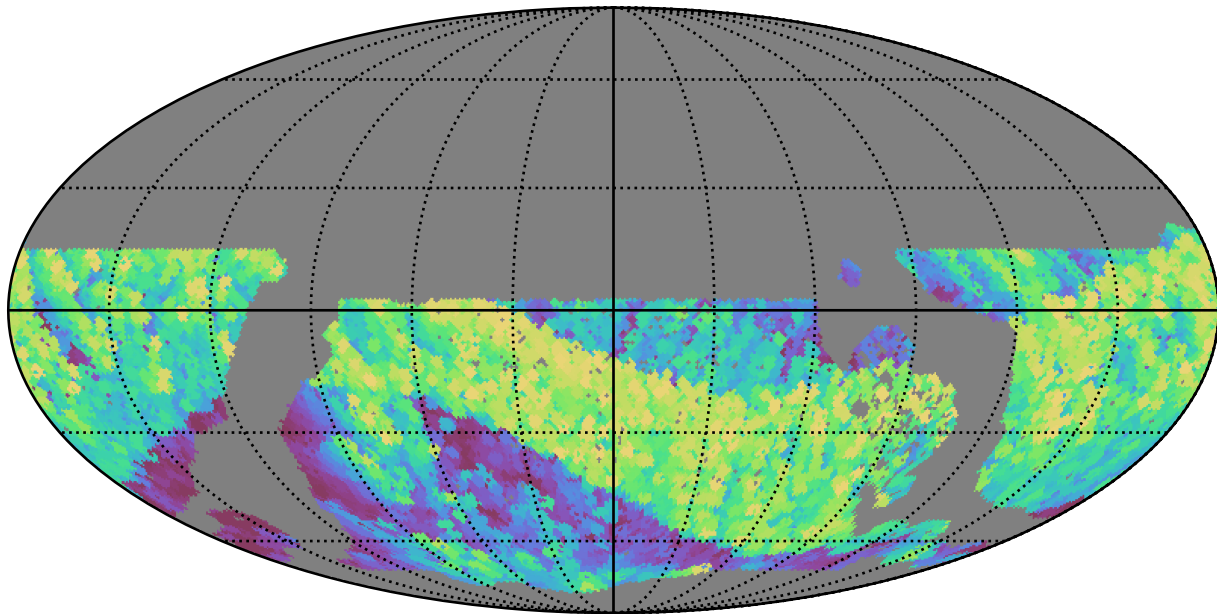
no_long_daily_v3.4_10yrs WFD z band: Max airmass
