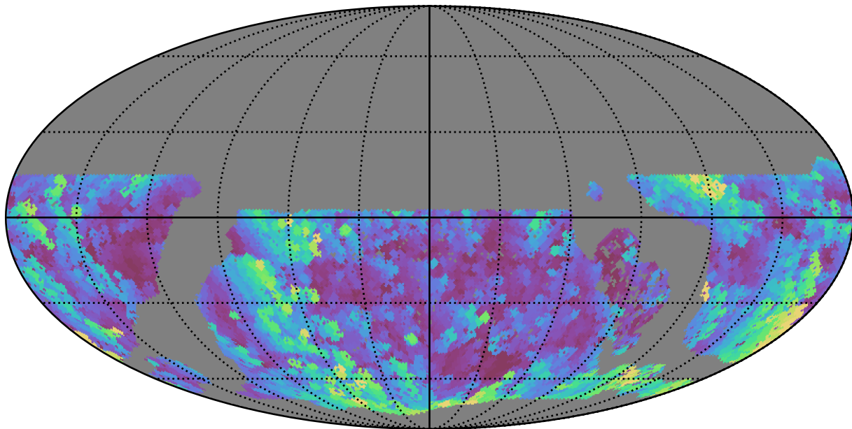
no_long_daily_v3.4_10yrs WFD u band: Max airmass
