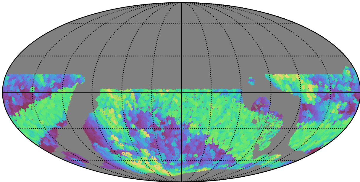
no_long_daily_v3.4_10yrs WFD r band: Max airmass
