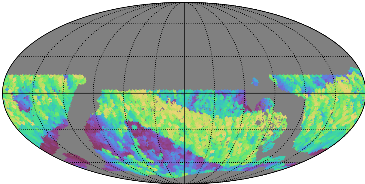
no_long_daily_v3.4_10yrs WFD i band: Max airmass
