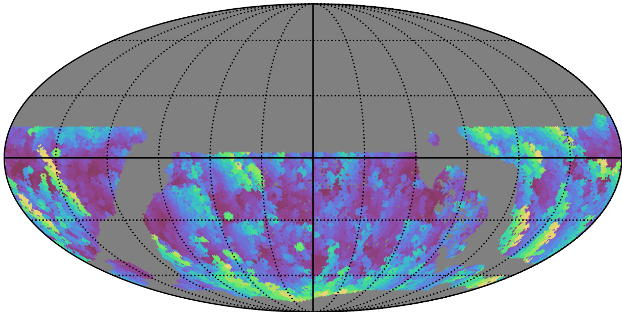
no_long_daily_v3.4_10yrs WFD g band: Max airmass
