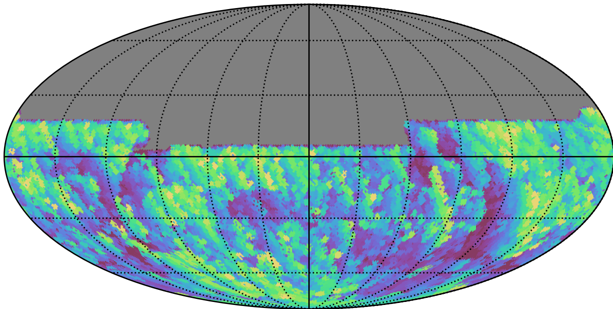
no_long_daily_v3.4_10yrs All sky y band: Max airmass
