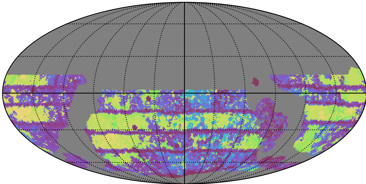
no_long_daily_v3.4_10yrs WFD y band: Max Inter-Night Gap
