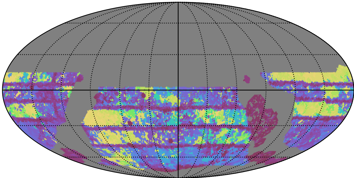
no_long_daily_v3.4_10yrs WFD i band: Max Inter-Night Gap
