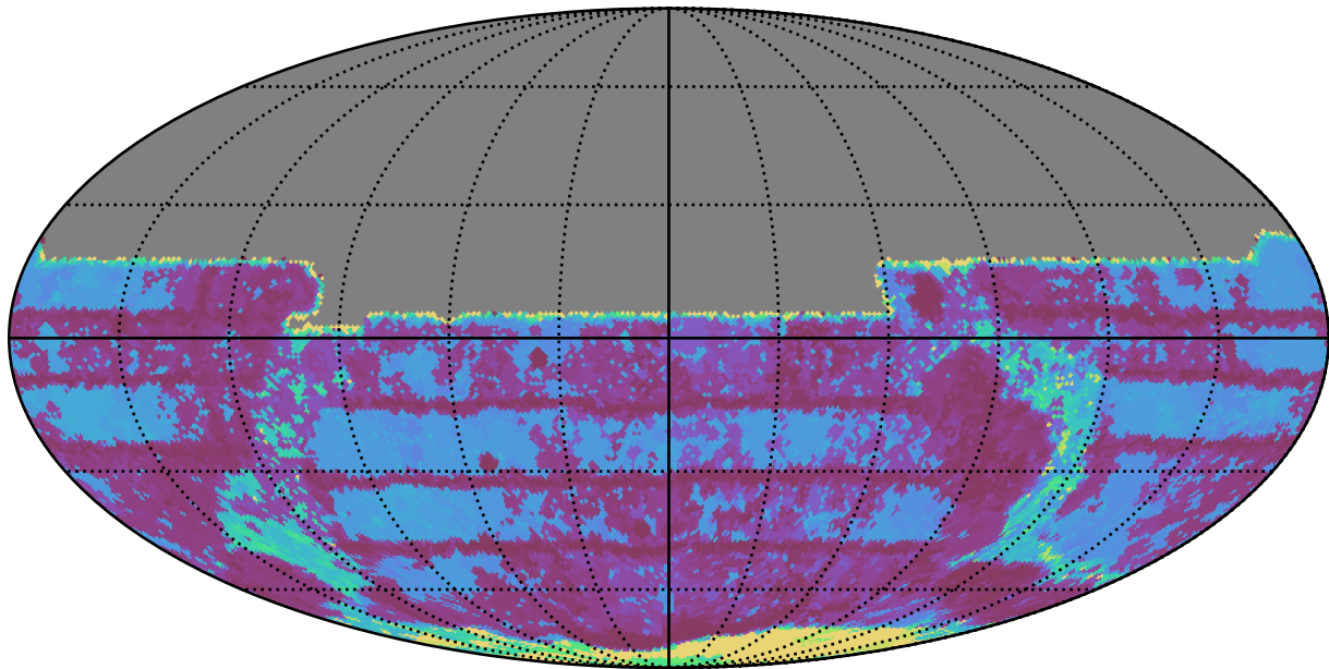
no_long_daily_v3.4_10yrs All sky y band: Max Inter-Night Gap
