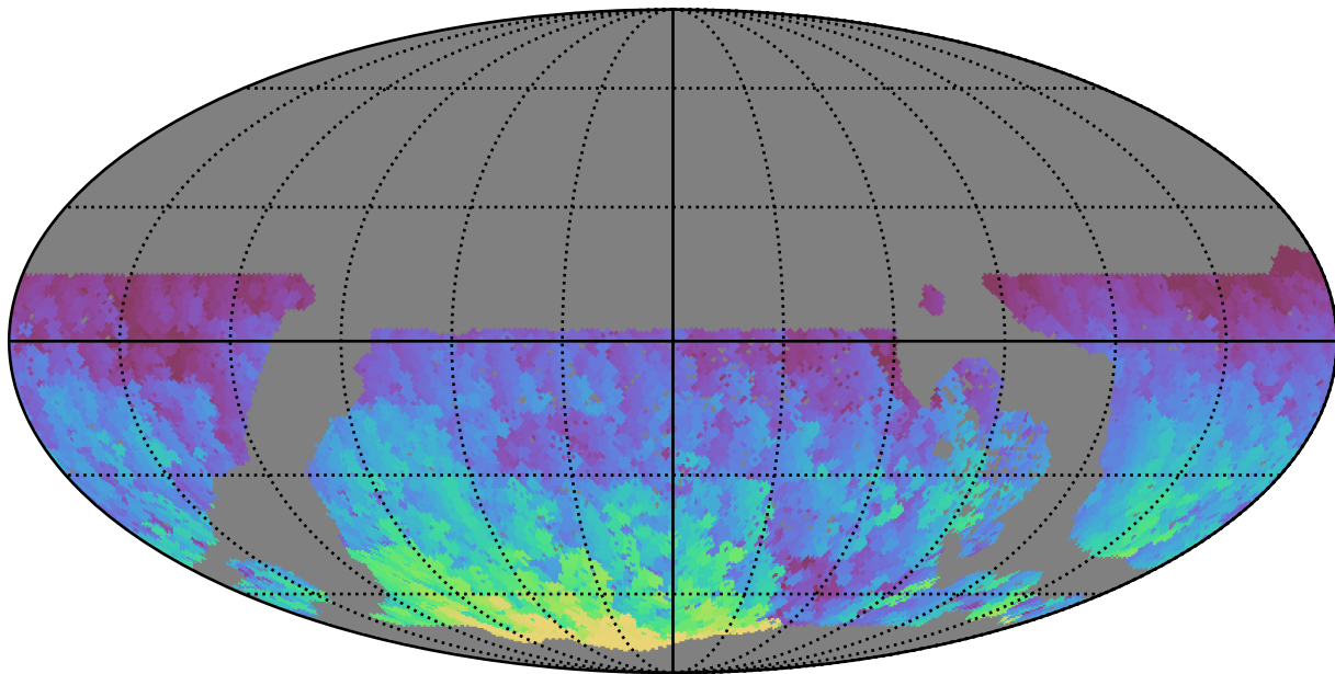
no_long_daily_v3.4_10yrs WFD y band: Max HA
