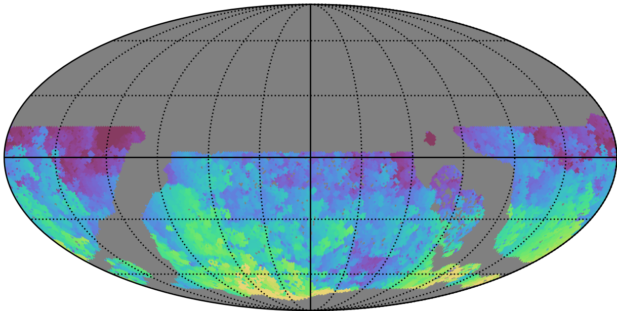
no_long_daily_v3.4_10yrs WFD u band: Max HA
