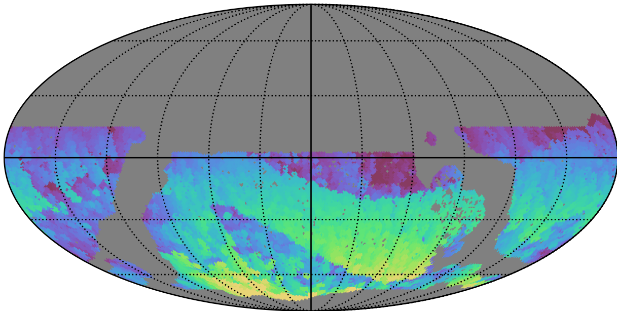
no_long_daily_v3.4_10yrs WFD i band: Max HA
