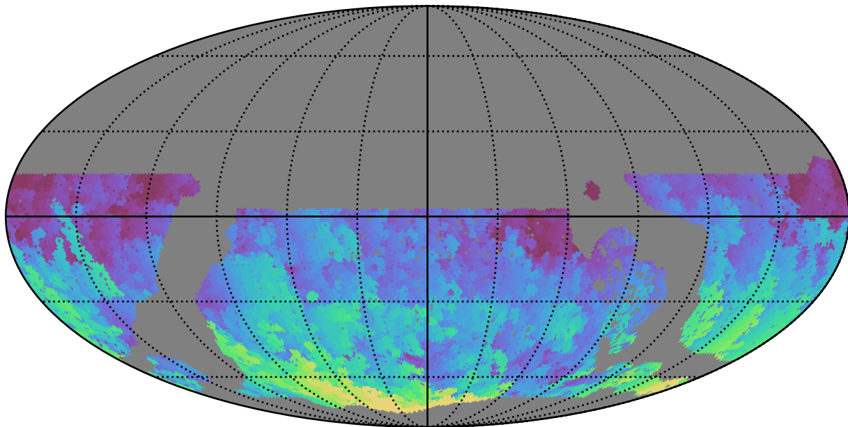
no_long_daily_v3.4_10yrs WFD g band: Max HA
