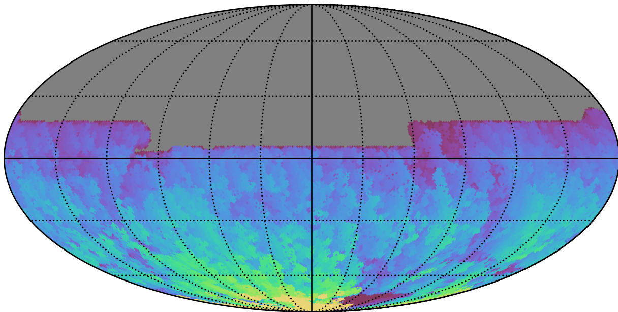
no_long_daily_v3.4_10yrs All sky y band: Max HA
