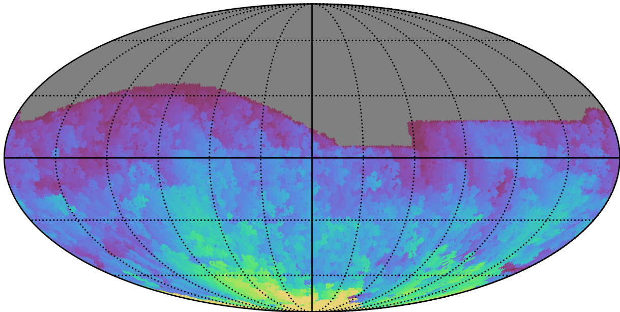
no_long_daily_v3.4_10yrs All sky r band: Max HA
