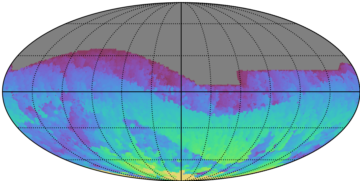
no_long_daily_v3.4_10yrs All sky i band: Max HA
