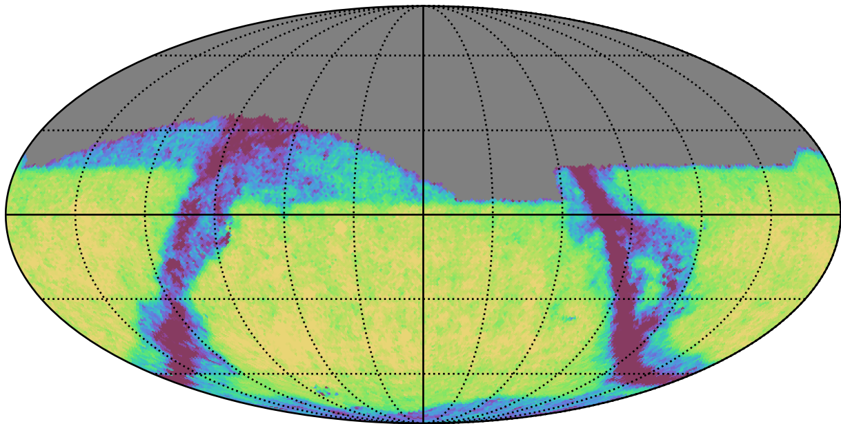
no_long_daily_v3.4_10yrs Yr 1 z band: Exgal_CoaddM5
