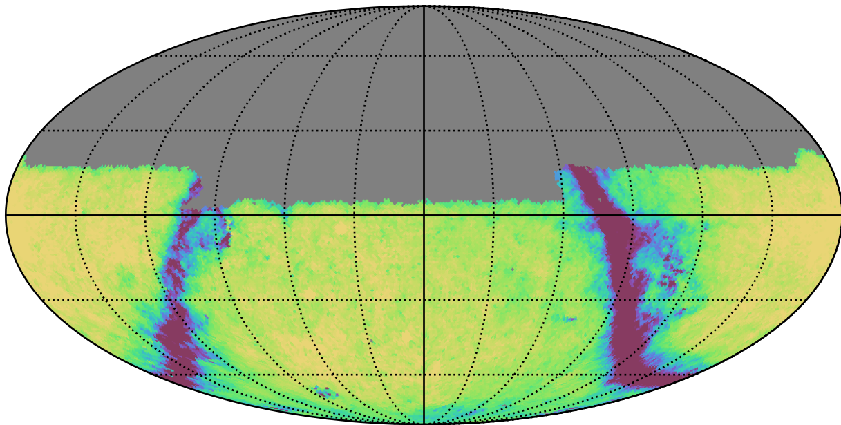
no_long_daily_v3.4_10yrs Yr 1 u band: Exgal_CoaddM5
