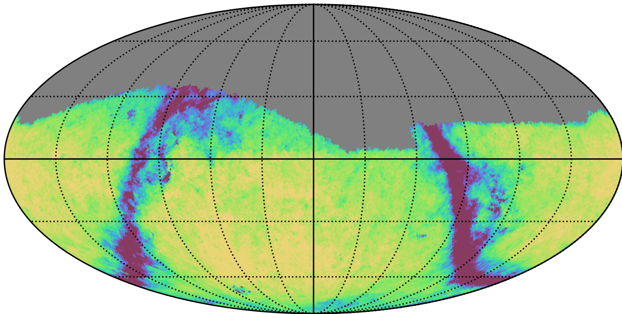
no_long_daily_v3.4_10yrs Yr 1 g band: Exgal_CoaddM5
